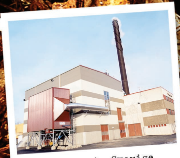
Tranås Energi, Sverige 1,8 MWe/ 10 MWth
