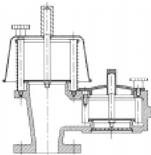
tryck-/vakuumentil
